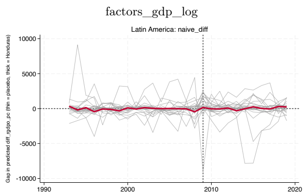
naive_diff
