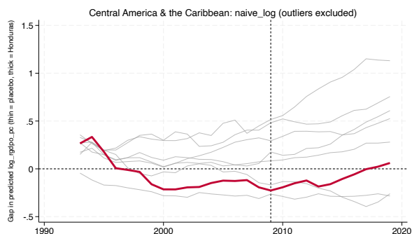
naive_log
