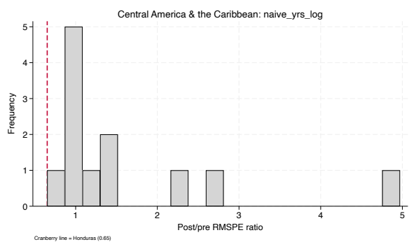
naive_yrs_log
