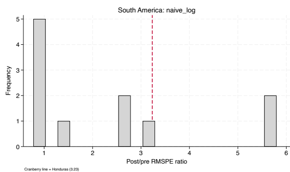
naive_log
