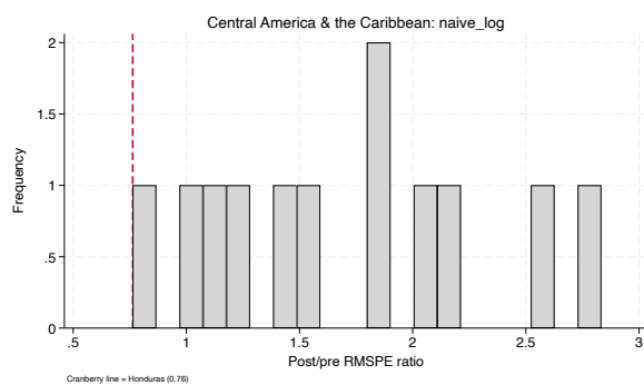
naive_log
