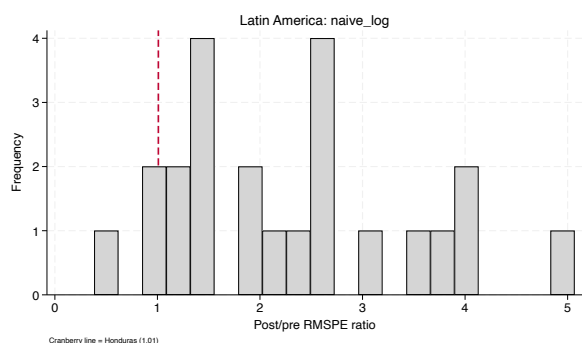
naive_log
