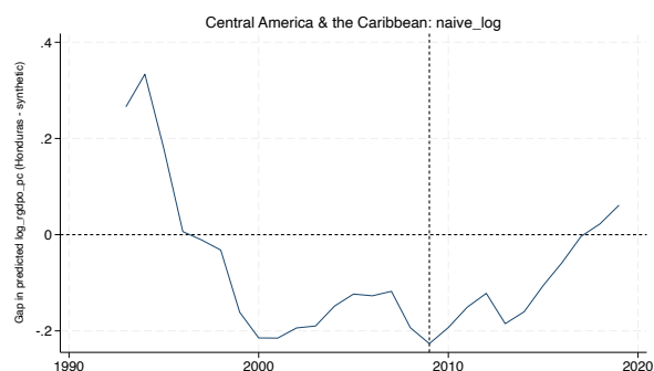
naive_log
