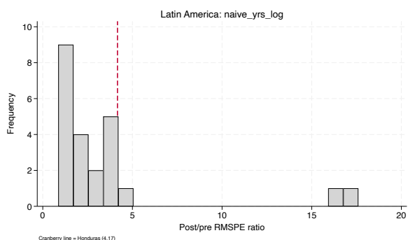
naive_yrs_log
