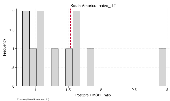
naive_diff
